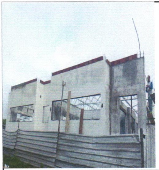
FOTO - 04 - ALVENARIA DE VEDAÇÃO COM ELEMENTO VAZADO DE CERÂMICA(COBOGÓ)
