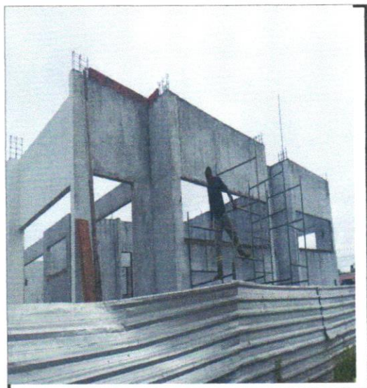
FOTO - 07 - ALVENARIA DE VEDAÇÃO DE BLOCOS CERÂMICOS FURADOS NA VERTICAL DE 14X19X39CM (ESPESSURA 14CM) DE PAREDES
