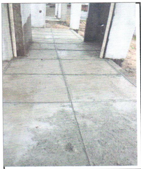
FOTO - 19 - Passeio em concreto desempenado com junta plastica a cada 1,20m espessura 10cm
