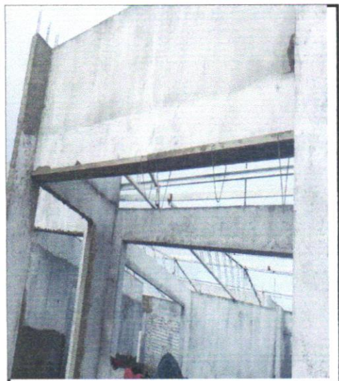
FOTO - 03 - ALVENARIA DE VEDAÇÃO DE BLOCOS CERÂMICOS FURADOS NA VERTICAL DE 14X19X39CM (ESPESSURA 14CM) DE PAREDES
