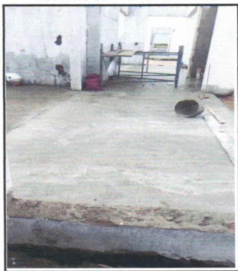
FOTO - 01 - CONTRAPISO EM ARGAMASSA TRAÇO 1:4 (CIMENTO E AREIA), PREPARO MECÂNICO COM BETONEIRA 400 L
