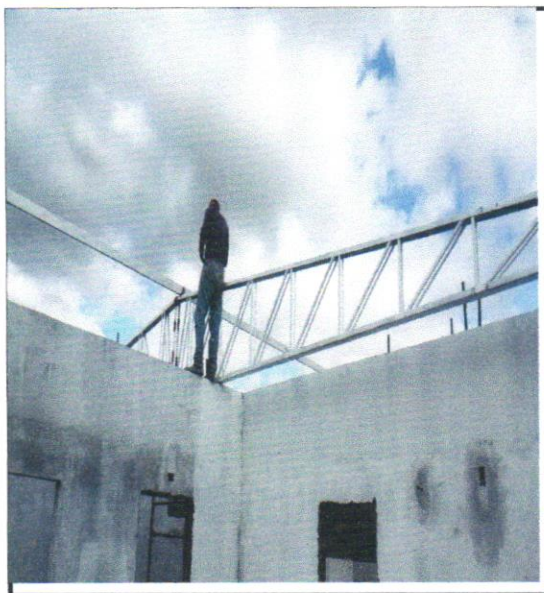
FOTO - 30 - TRAMA DE AÇO COMPOSTA POR TERÇAS PARA TELHADOS DE ATÉ 2 ÁGUAS PARA TELHA
