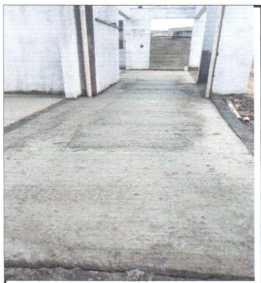
FOTO -13 - CONTRAPISO EM ARGAMASSA TRAÇO 1:4 (CIMENTO E AREIA), PREPARO MECÂNICO COM BETONEIRA 400 L, APLICADO
