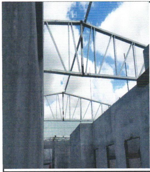
FOTO - 28 - TRAMA DE AÇO COMPOSTA POR TERÇAS PARA TELHADOS DE ATÉ 2 ÁGUAS PARA TELHA
