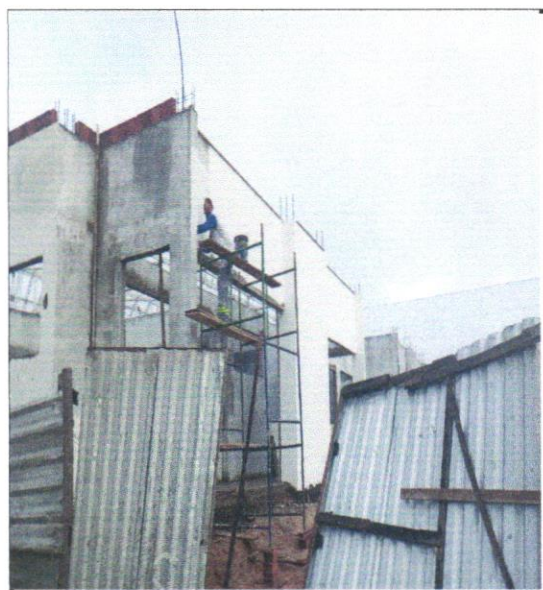
FOTO - 24 - APLICAÇÃO MANUAL DE MASSA ACRÍLICA EM PANOS DE FACHADA
