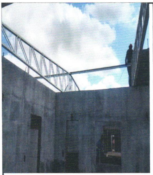
FOTO - 29 - TRAMA DE AÇO COMPOSTA POR TERÇAS PARA TELHADOS DE ATÉ 2 ÁGUAS PARA TELHA
