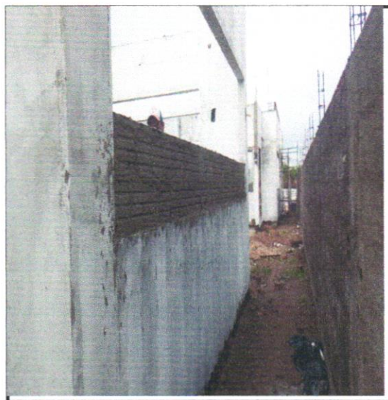
FOTO - 16 - EMBOÇO OU MASSA ÚNICA EM ARGAMASSA TRAÇO 1:2:8, PREPARO MECÂNICO
