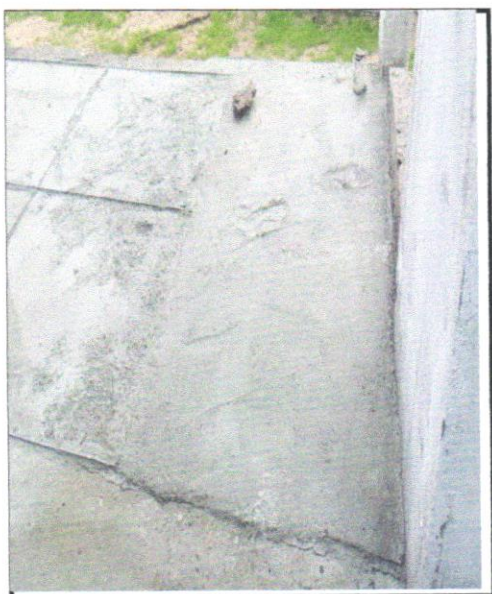
FOTO - 17 - Passeio em concreto desempenado com junta plastica a cada 1,20m espessura 10cm
