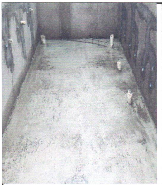
FOTO - 21 - CONTRAPISO EM ARGAMASSA TRAÇO 1:4 (CIMENTO E AREIA), PREPARO MECÂNICO COM BETONEIRA 400 L, APLICADO
