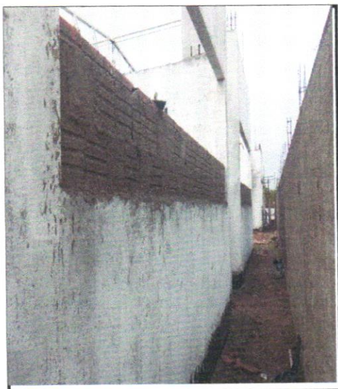
FOTO - 09 - EMBOÇO OU MASSA ÚNICA EM ARGAMASSA TRAÇO 1:2:8, PREPARO MECÂNICO
